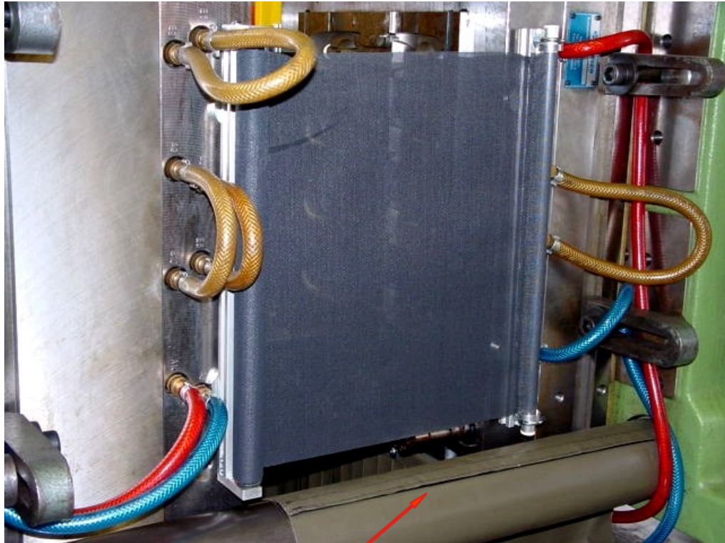
Holmabdeckung mit Klettverschluss und Ausfallrutsche.
